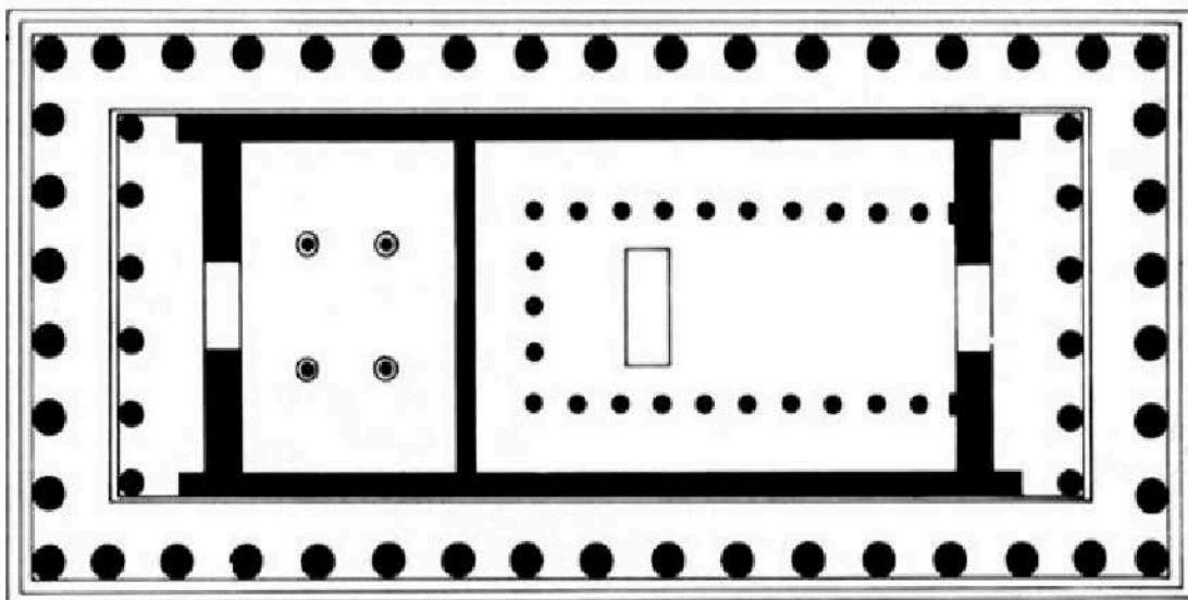
2. El Partenón.
